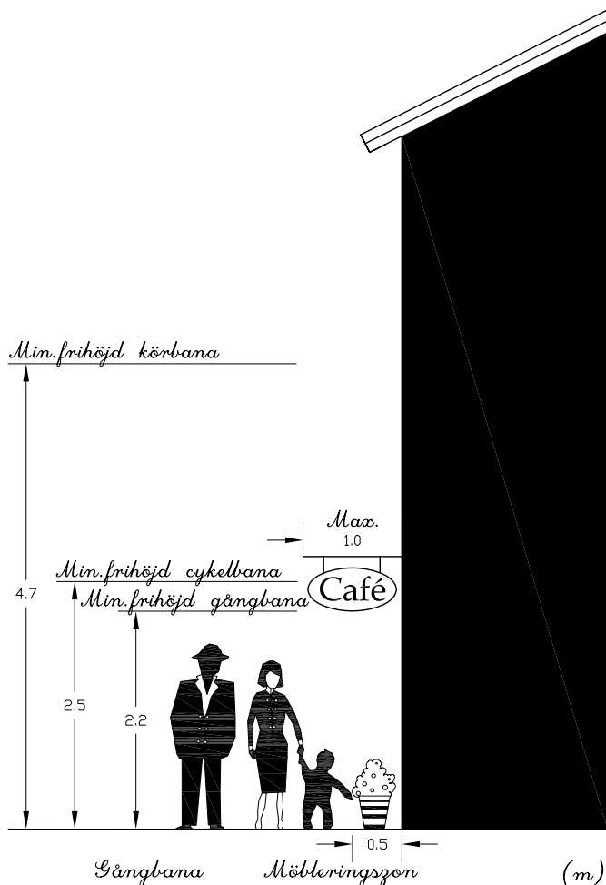
Principsektionen visar möbleringszonen samt frihöjderna för konsolmonterade skyltar.
